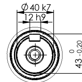
DETTAGLIO A
